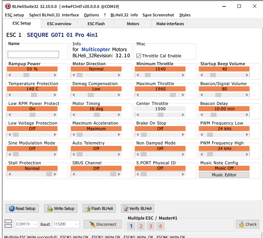
BLHeli_32固件可视化编程调参界面
